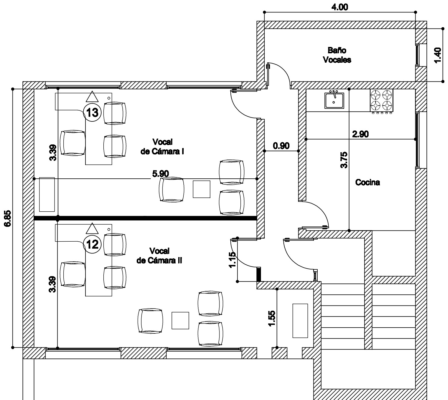
Planta Alta Superficie: 90 m 2
