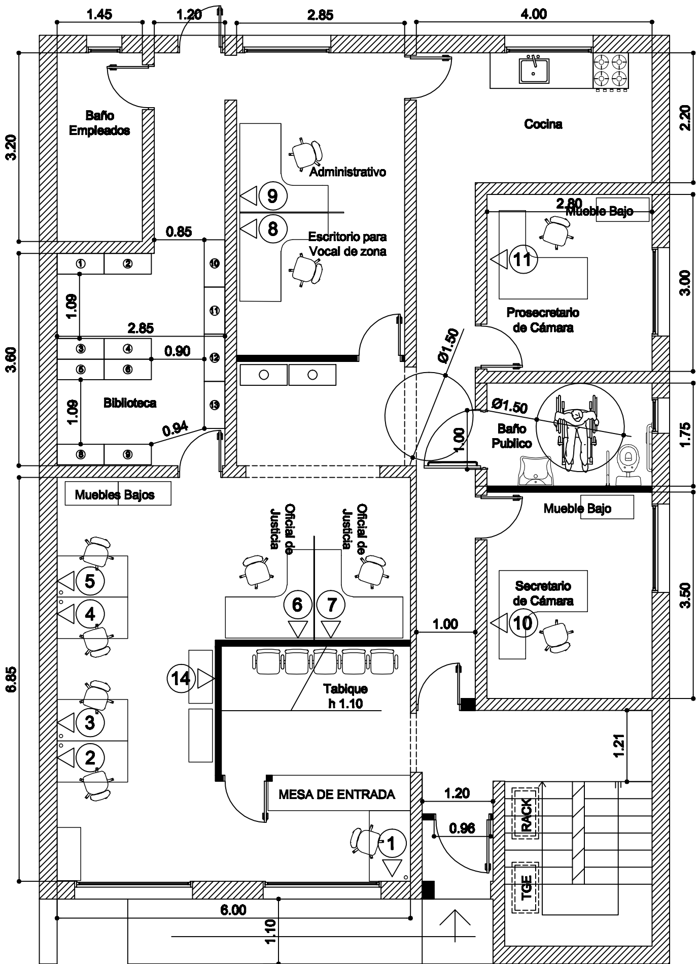
Planta Baja Superficie: 163 m 2
